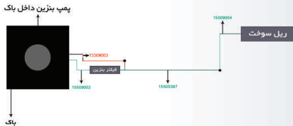
سیستم سوخت رسانی سمند دنا ( مدل ۹۴ به بالا )
