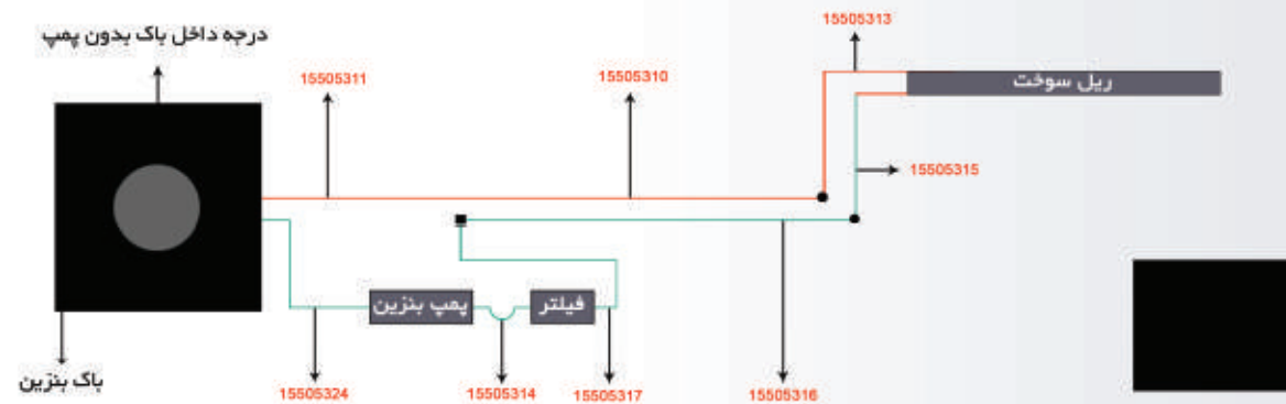
سیستم سوخت رسانی این لاین ۴۰۵ ( XU7 ) مدل ۸۰ - ۸۱ - ۸۲
