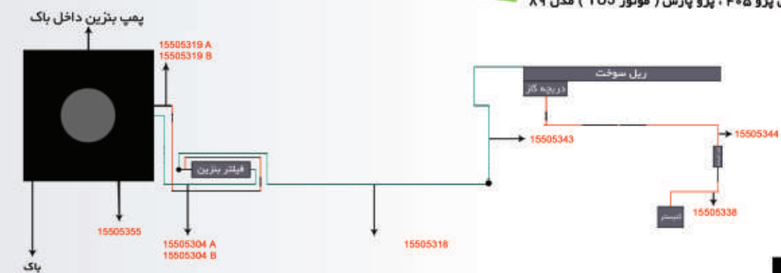
سیستم سوخت رسانی پژو ۴۰۵ ، پژو پارس ( موتور TU5 ) مدل ۸۹
