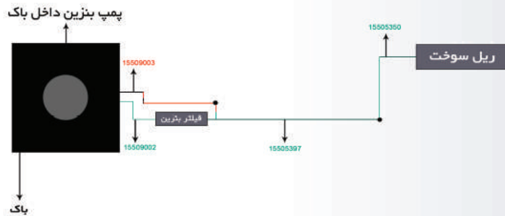
سیستم سوخت رسانی این لاین ( EF7 ) مدل ۹۴ به بالا
