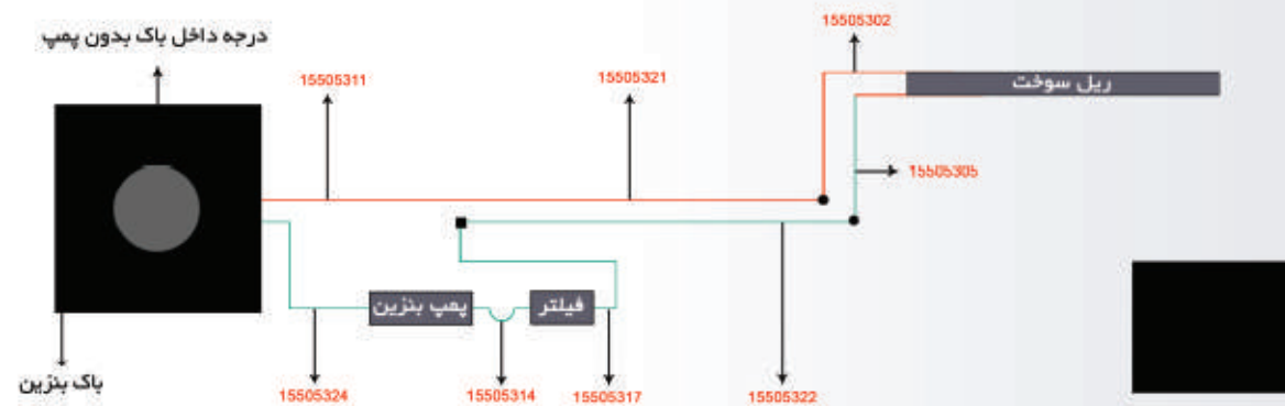
سیستم سوخت رسانی این لاین ۴۰۵ ( XU7 ) مدل ۸۳
